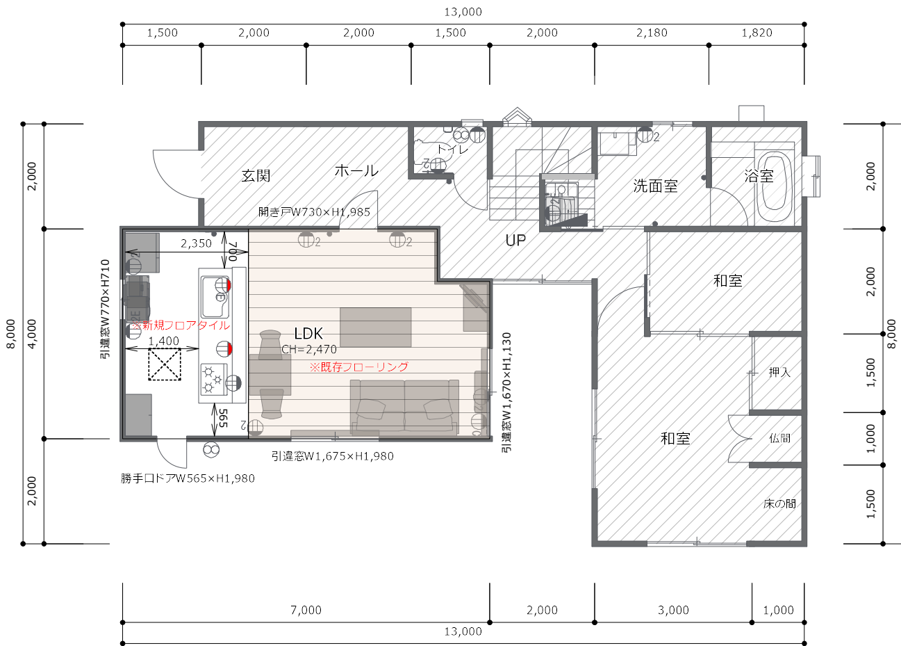
リフォーム後平面図 S = 1 / 100
