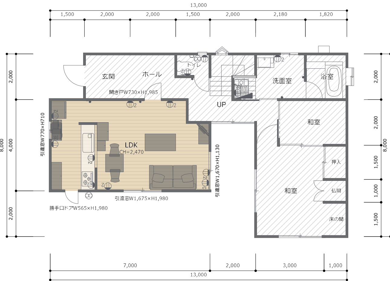
既存1F平面図 S = 1 / 100
